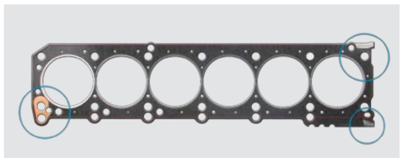
Figura 2_Nuevo modelo 61-28975-30
