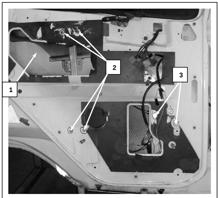
Puerta lado izquierdo, Portière avant gauche, Left front door, Porta frente esquerda
