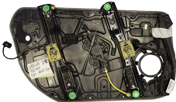
Elevallunas original / OEM window regulator / Lève-vitre original / Elevador de vidro original
