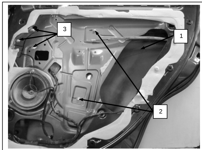
Puerta lado derecho, Portière arrière droite, Right rear door, Porta traseira direita
