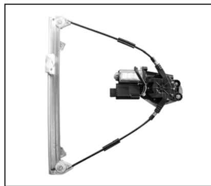
Nuestro elevavinas – notre lève-vitre – our window regulator – nosso levantador de vidro
