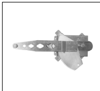
Nuestro elevallas – notre lève-vitre – our window regulator – nosso levantador de vidro
