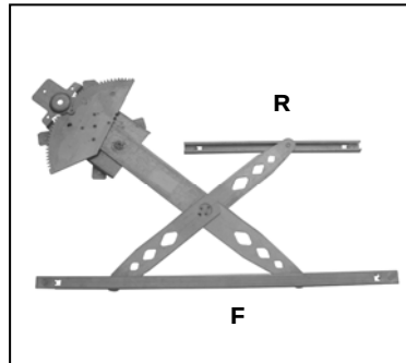
Nuestro elevallunas – notre lève-vitre – our window regulator – nosso levantador de vidro
