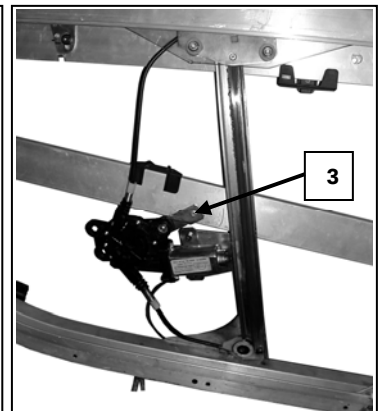
Puerta lado izquierdo, Portière avant gauche, Left front door, Porta frente esquerda
