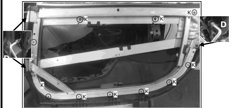
Puerta lado izquierdo, Portière avant gauche, Left front door, Porta frente esquerda
