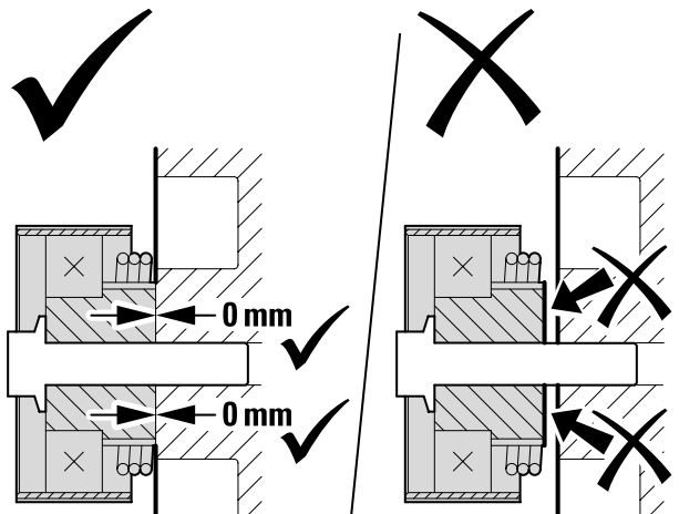
Figura 2: Stânga – Rola întinzătorului este în contact cu întreaga suprafață de montare a sa pe motor. Dreapta – Rola întinzătorului nu este în contact cu întreaga suprafață de montare a sa pe motor.
