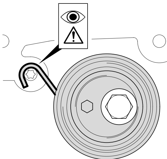
Figura 1: Montarea corectă a arcului pe bolțul său de ancorare
