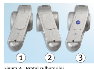
Figura 3: Brațul culbutorilor
