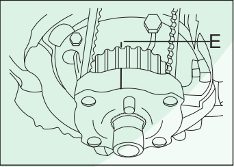
FIGURA 5 Verificar la correcta alineación de las marcas de puesta en fase E.
