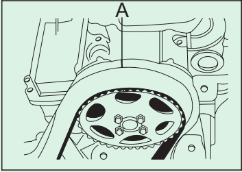
FIGURA 1 Verificar la correcta alineación de las marcas de puesta en fase A.
