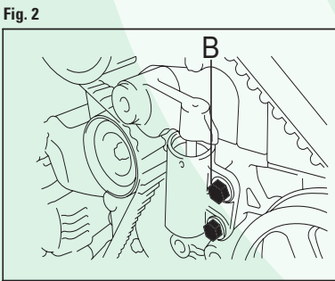
FIGURA 2 Aflojar los tornillos de fijación B del tensor de la correa, demónter les courroies de la distribución.
