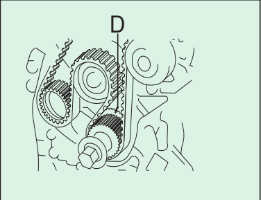
FIGURA 4 Controllare il corretto allineamento della tacca di fase D.
