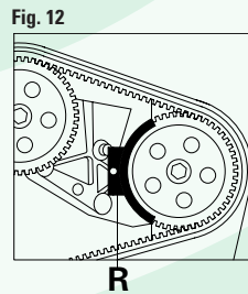
FIGURA 11 Controllare il corretto allineamento delle tacche di fase Q. FIGURA 12 Inserire l'apposito attrezzo di bloccaggio della puleggia della pompa di iniezione R.
