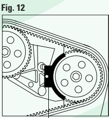
FIGURA 11 Verificar la correcta alineación de las marcas de fase Q. FIGURA 12 Insertar la herramienta para inmovilización de polea de bomba de inyección R.
