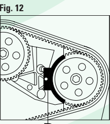
FIGURA 11 Controllare il corretto allineamento delle tacche di fase Q. FIGURA 12 Inserire l'apposito attrezzo di bloccaggio della puleggia della pompa di iniezione R.
