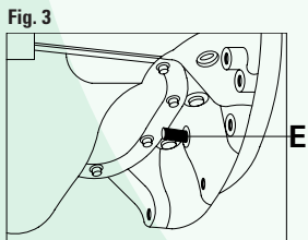
FIGURA 3 Inserire l'apposito attrezzo di bloccaggio del volano E. FIGURA 4 Ruotare l'albero motore fino ad allineare il foro per la messa in fase del motore ed installare, quindi, l'apposito attrezzo di bloccaggio F.
