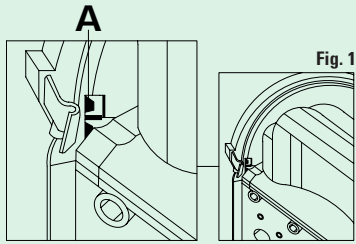
FIGURA 1 Verificar la correcta alineación de la marca de puesta a punto A.
